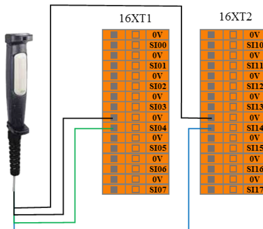
图 8-10 三态开关输入连接示意图
