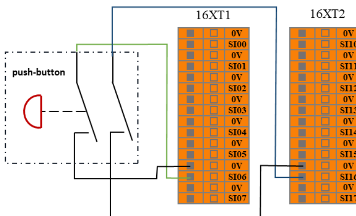
图 8-12 拖动示教输入连接示意图
