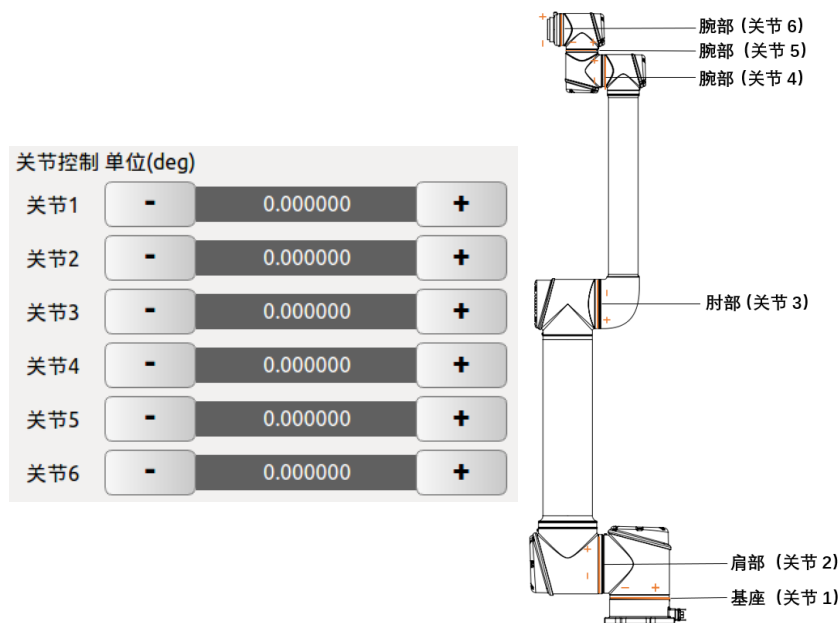
图 10-17 关节控制示意图
