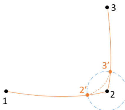
图 11-33 提前到达交融半径 Move J-Move J 运行轨迹示例
