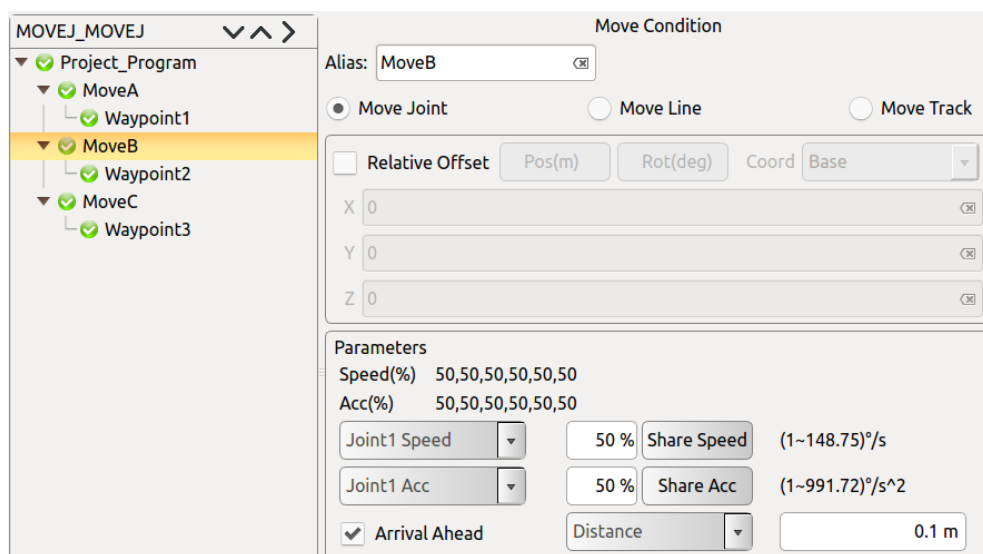
图 11-30 提前到达距离/时间 Move J-Move J 编程示例
