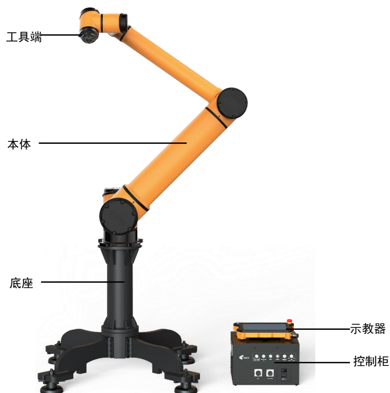
图 5-1 AUBO-i20 机器人系统
