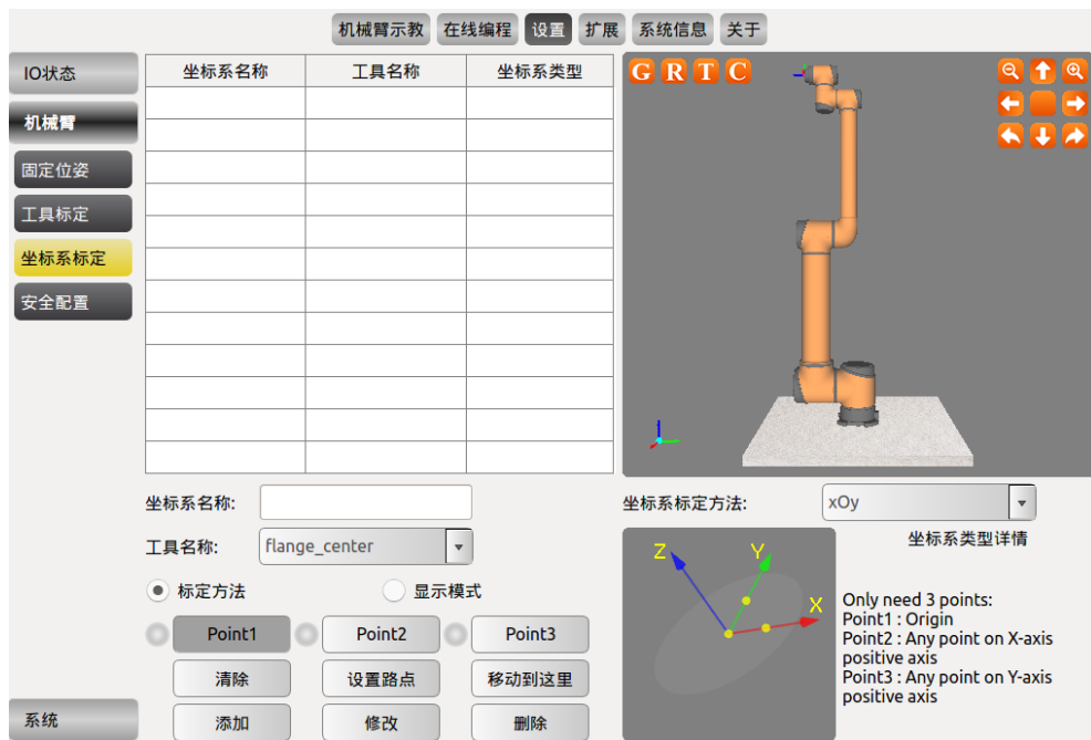
图 10-38 坐标系标定
