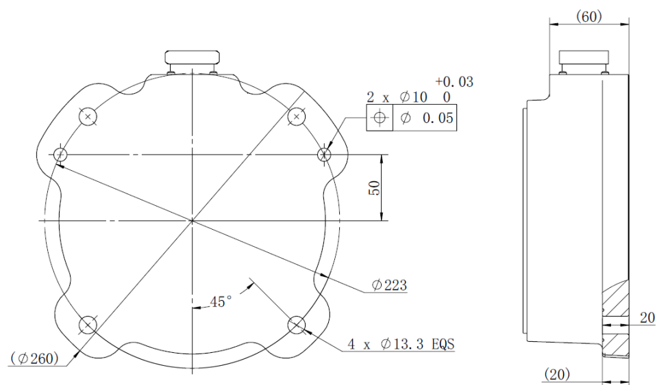
图 6-6 底座上的安装孔尺寸，单位为 mm
