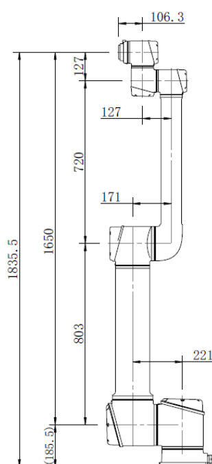
图 6-1AUBO-i20 机器人机械尺寸图（单位：mm）
