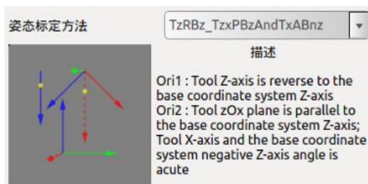
图 10-34 TzRBz_TzxPBzAndTxABnz
