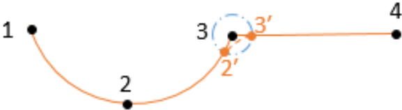
图 11-41 提前到达交融半径 Move arc-Move L 运行轨迹示例
