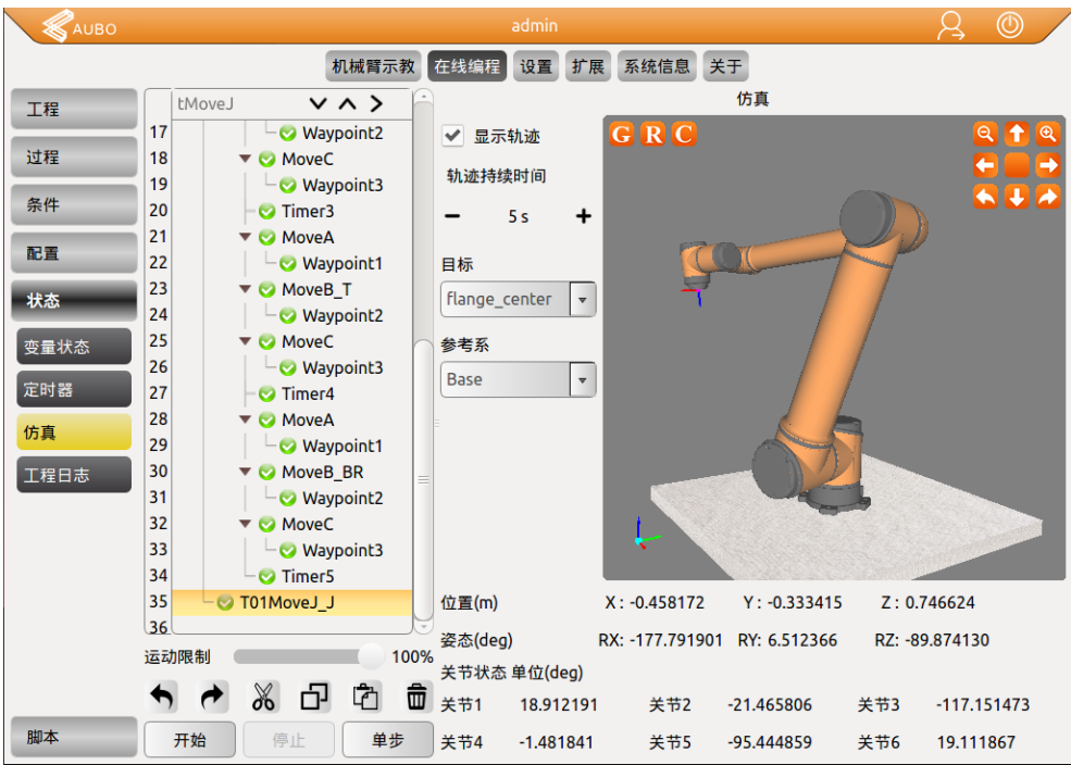
图 11-72 仿真模型
