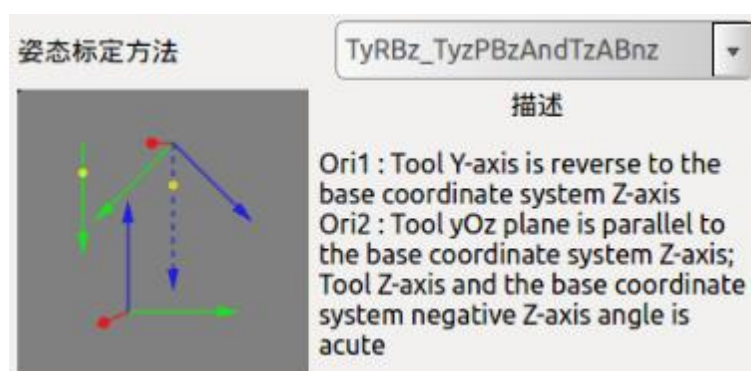
图 10-33 TyRBz_TyzPBzAndTzABnz
